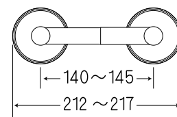
⑤P0610F(C) / ペーパーホルダー (フタ付き)
