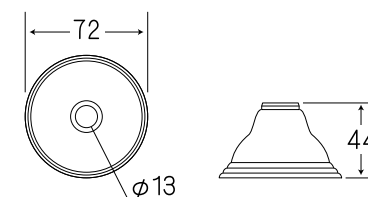
各アイテム共通 エスカッション
