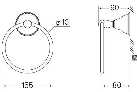
⑥P0611(C) / タオルリング
