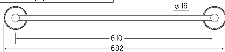
②P0608(C)-24" / タオルバー
