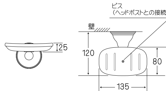
⑧P0613(C) / ソープディッシュ
