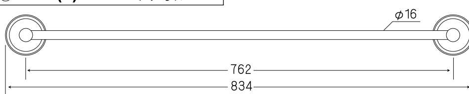
③P0609(C)-WP-30” / タオルバー
