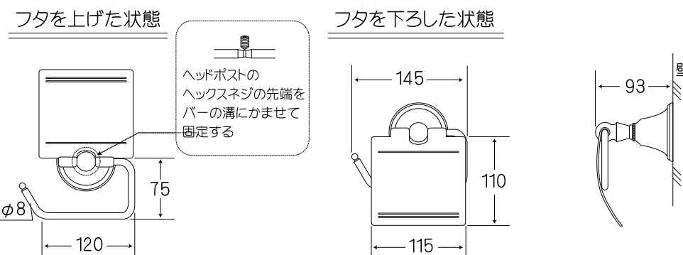
⑤P0610F(C)-WP / ペーパーホルダー (フタ付き)
