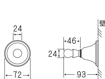
⑦P0612(C)-WP / ロープフック
