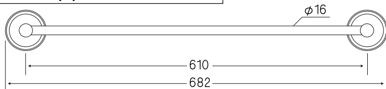
②P0608(C)-WP-24” / タオルバー
