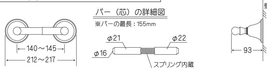
④P0610(C)-WP / ペーパーホルダー (フタ無)
