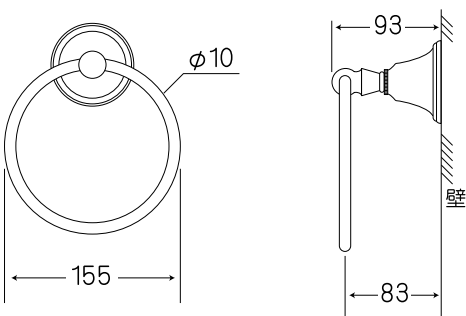
⑥P0611(C)-WP / タオルリング
