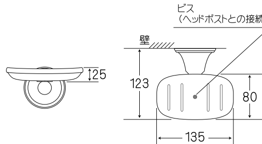
⑧P0613(C)-WP / ソープディッシュ
