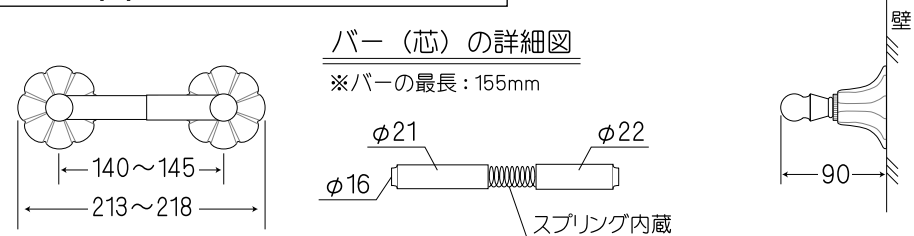
④P0507(C) / ペーパーホルダー (フタ無)
