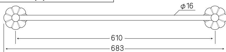
②P0504(C)-24" / タオルバー
