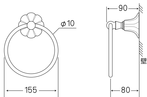
⑥P0510(C) / タオルリング
