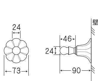
⑦P0508(C) / ロープフック
