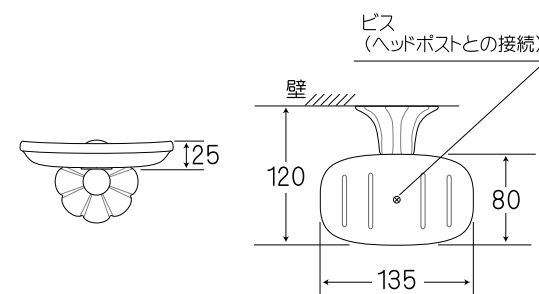
⑧P0506(C) / ソープディッシュ
