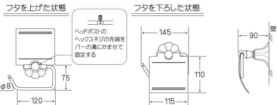
⑤P0507F(C) / ペーパーホルダー (フタ付き)
