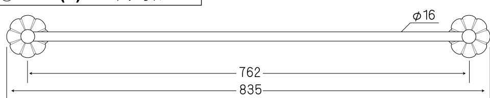
③P0505(C)-30" / タオルバー
