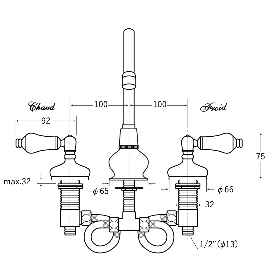
水栓金具取付穴
