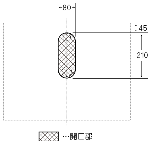
カウンター開口寸法の目安 (排水ドレインHL-4534 使用の場合)
