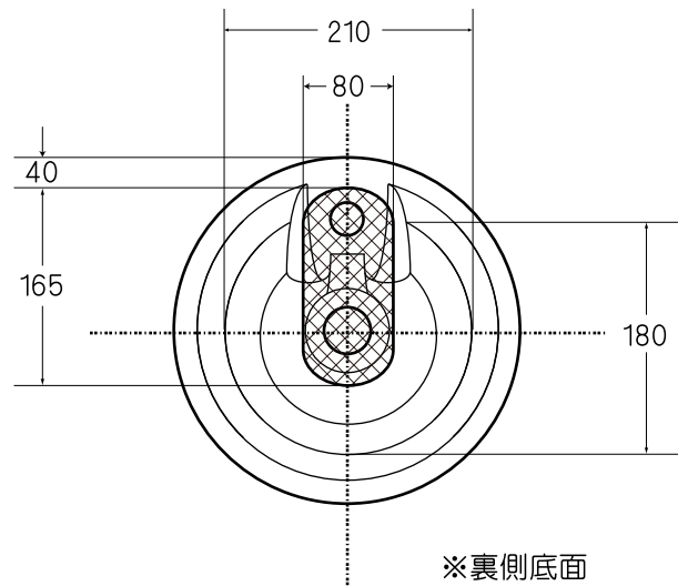
カウンター開口寸法を目安 （水栓金具 #20001,HL-4534 使用の場合）
