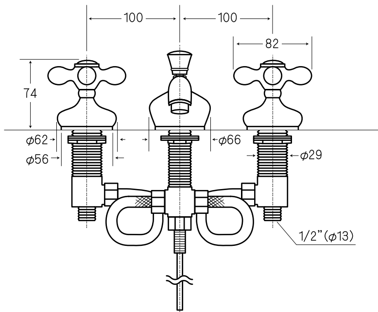
水栓金具取付穴
