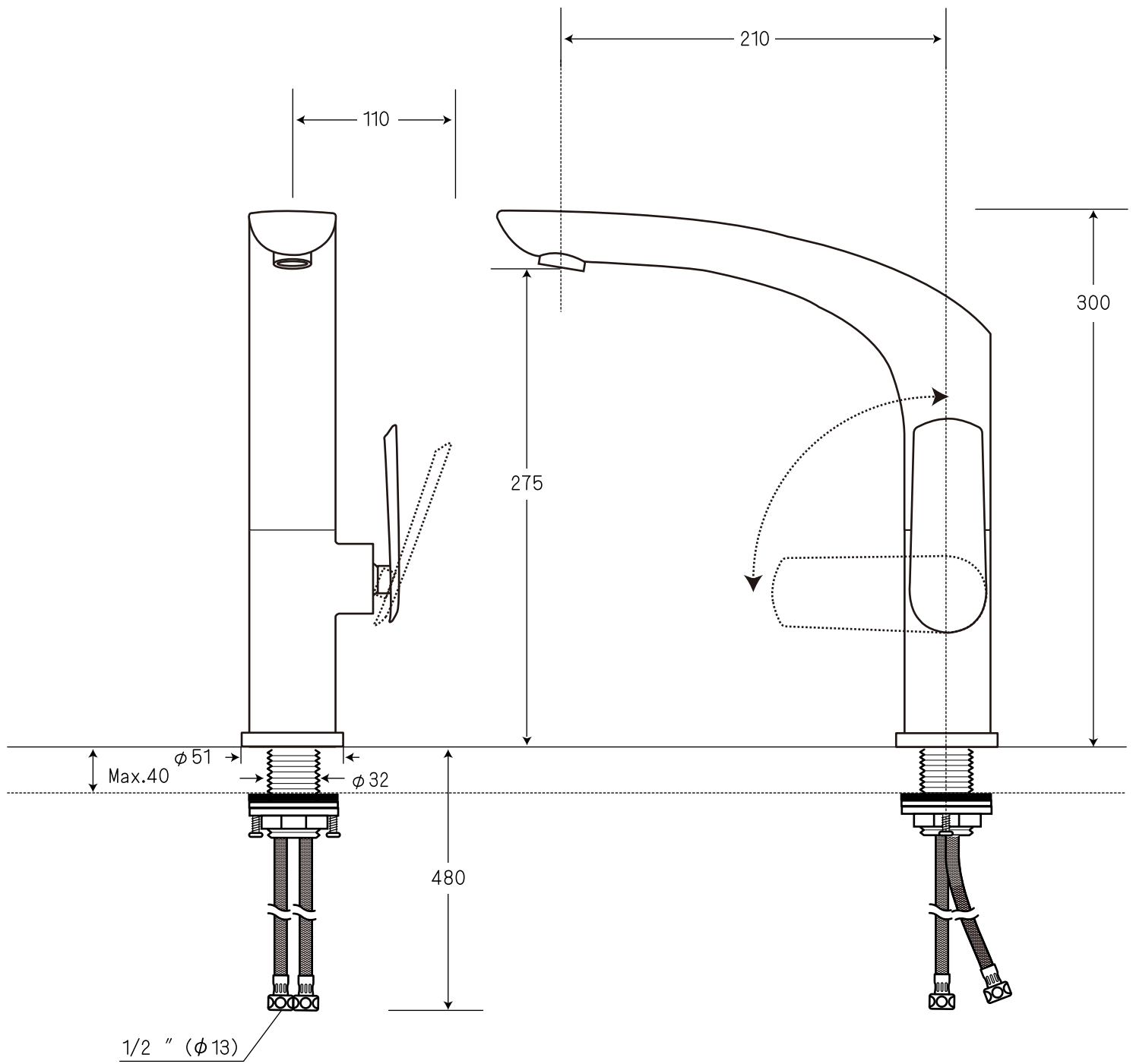
水栓金具取付穴
